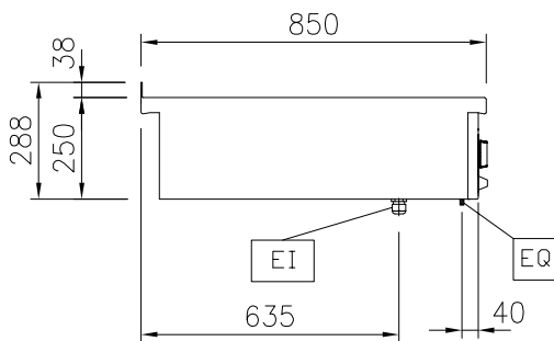
Zij aanzicht
