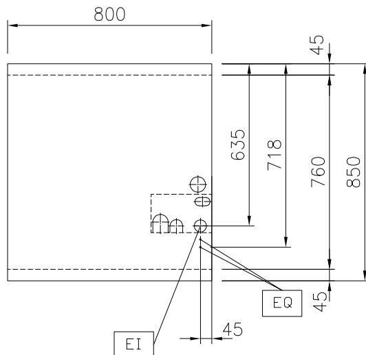
Boven aanzicht
